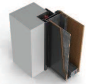
Estructuras de 86 mm espesor totalmente en acero galvanizado con sistema de cierre de 3 y 5 puntos.
